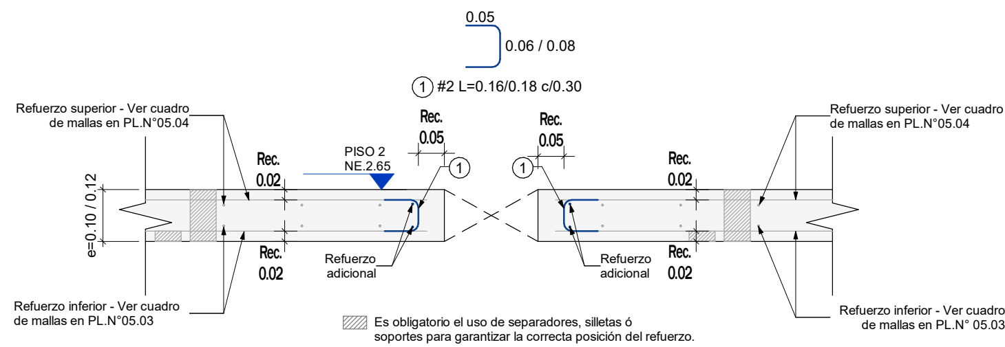
DETALLE TÍPICO - UBICACIÓN REFUERZO ADICIONAL Escala 1 : 10
