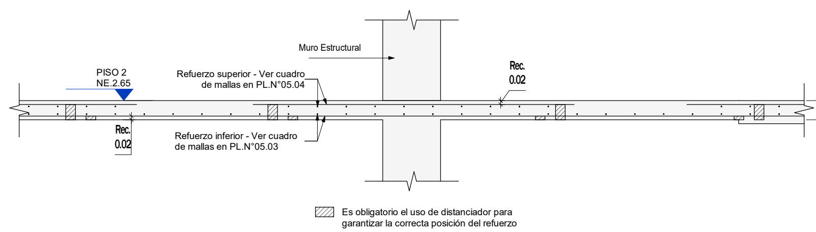
CORTE TÍPICO PLACA ÁEREA e=0.10 Escala 1 : 20
