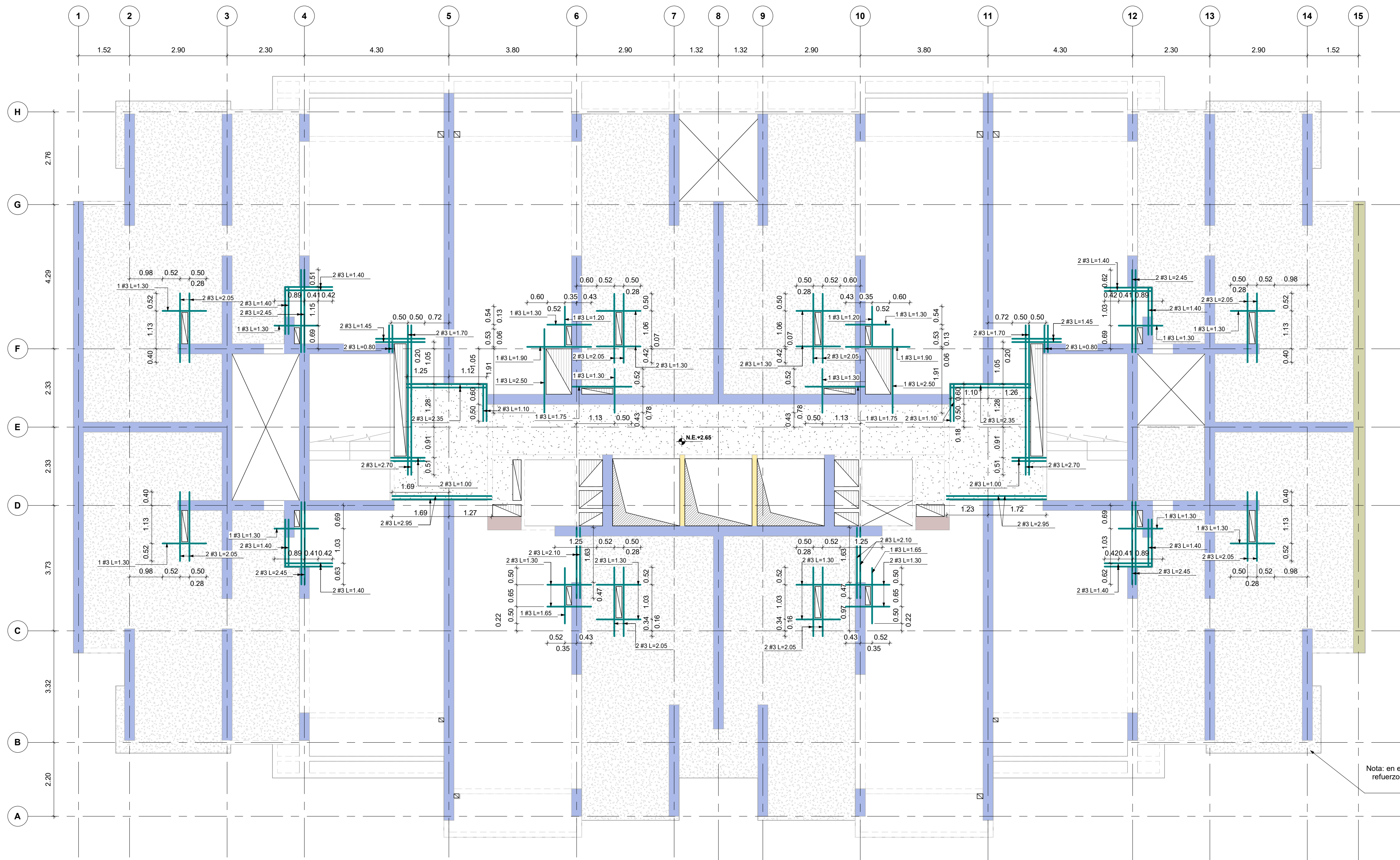
PLANTA DE REFUERZO ADICIONAL (INFERIOR Y SUPERIOR) PISO 2 Escala 1 : 75
