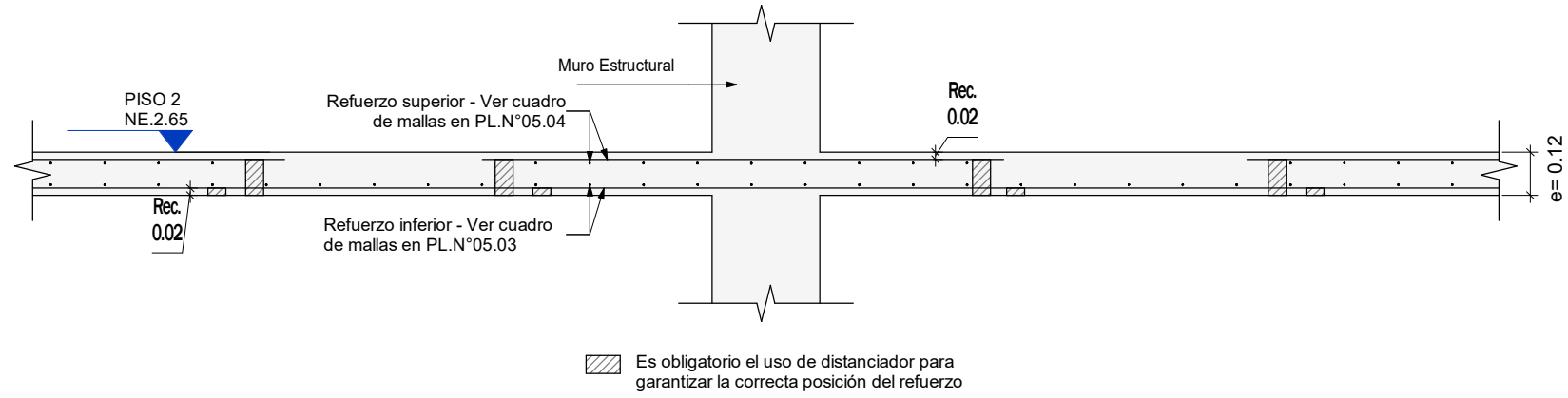
CORTE TÍPICO PLACA ÁEREA e=0.12 Escala 1 : 20
