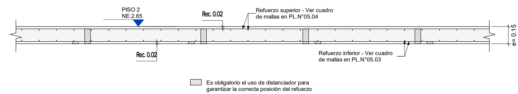
CORTE TÍPICO PLACA ÁEREA e=0.15 Escala 1 : 20
