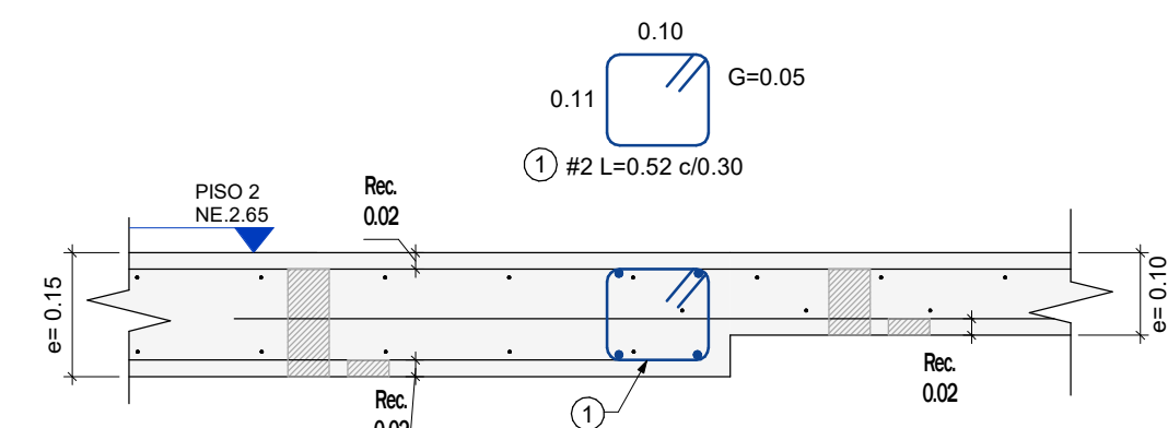
DETALLES TÍPICOS - CAMBIO DE SECCIÓN Escala 1 : 10
